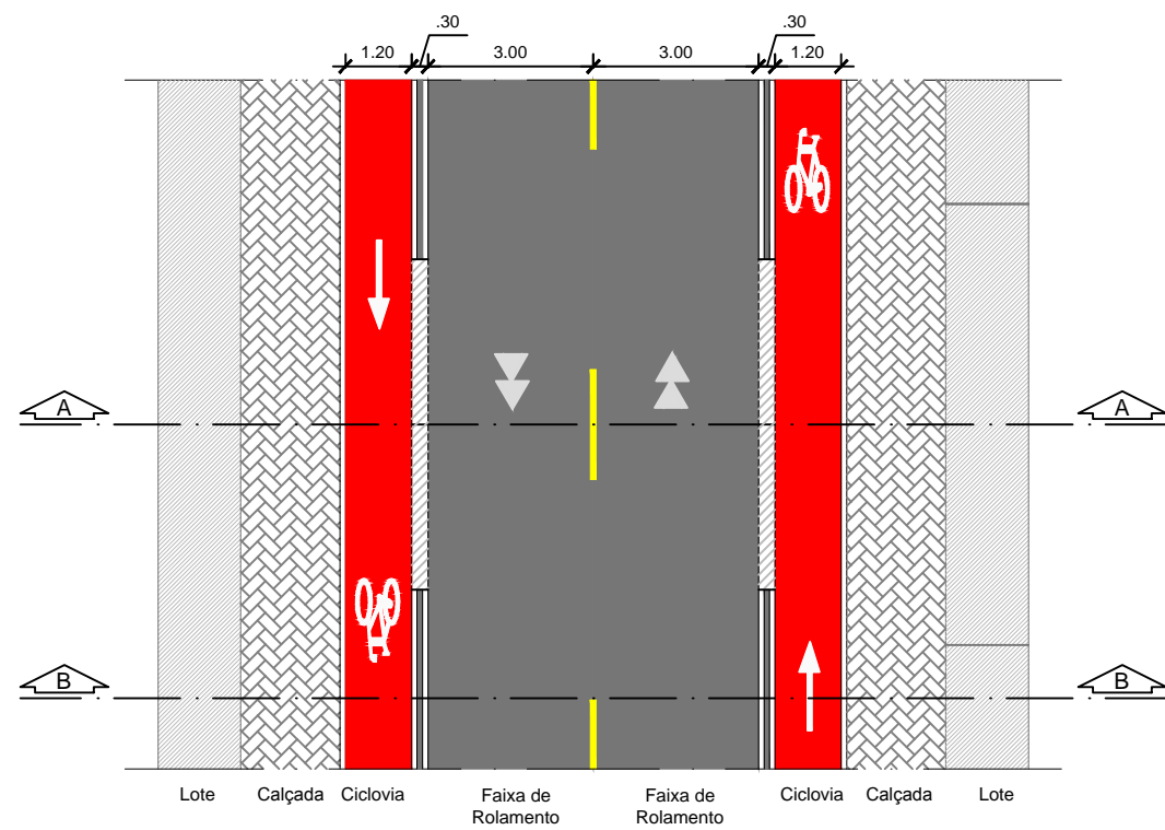
PLANTA TIPOLOGIA 1
